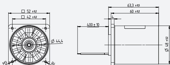
Micronel Tube Fan D483P-024KM-4
