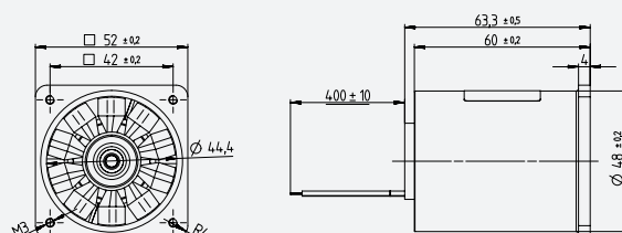
Micronel Tube Fan D484P-024KM-4
